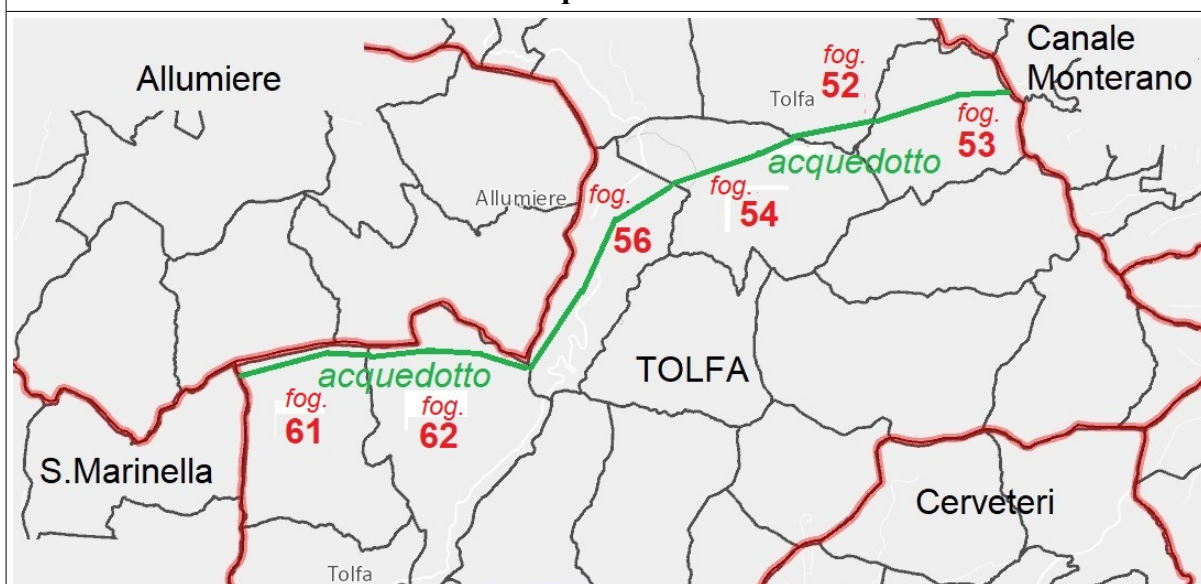
FIG. 2 – tracciato dell'acquedotto
